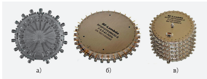
Рис. 25. Конструкции многопозиционных дисковых переключателей: а – SP10Т (KA-2060-LK, Kratos); б – SP32Т (RFSP32TA5M43G-S, RF-Lambda); в – SP160Т (RFSP160TA0020G-S, RF-Lambda)
