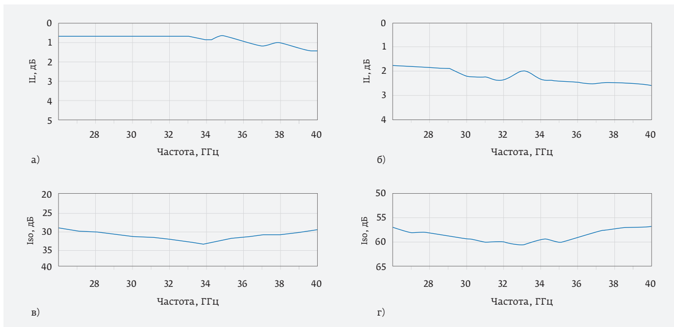
Рис. 36. Зависимости вносимых потерь IL (а, б) и развязки Iso (в, г) от частоты в волноводных SPST pin-переключателях HSW2801 (а, в) и HSW2803 (б, г), выпускаемых компанией НХИ
