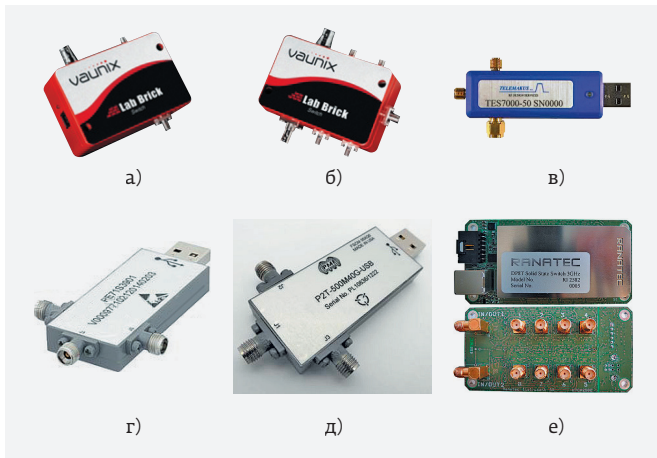
Рис. 33. Конструкции переключателей, программируемых по USB-интерфейсу: а – LSW-602PDT (Vaunix); б – LSW-602P4T (Vaunix); в – TES7000-50 (Telemakus); г – PE71S3901 (Pasternack); д – P2T-500M40G-USB (PMI); е – RI 2582 (Ranatec)
