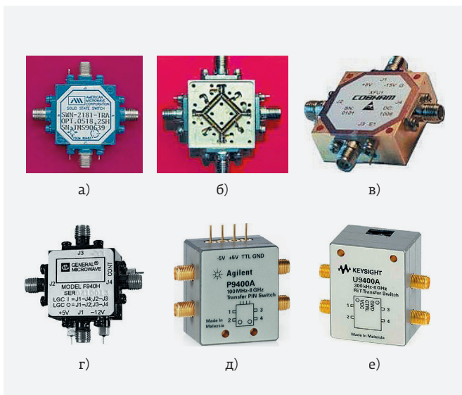
Рис. 30. Конструкции модульных DPDT-переключателей: а, б – модель SWN-2181-TRA (АМС) с верхней крышкой и без нее; в – модель XFU1 (Cobham Signal & Control Solutions); г – модель F940H (Kratos); д, е – модели P9400A и U9400A (Keysight)
