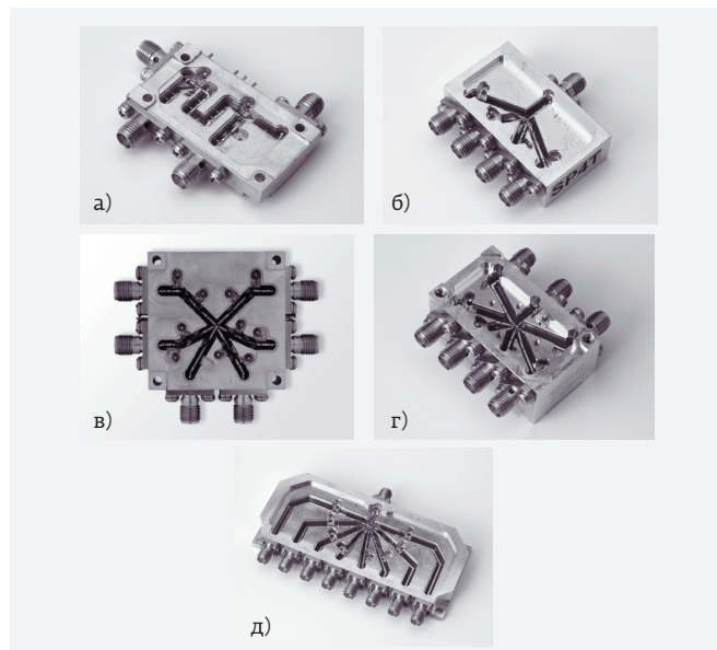
Рис. 20. Внутреннее устройство многопозиционных переключателей, выпускаемых компанией Elbit Systems: а – SP3Т (серия MW123Т); б – SP4Т (серия MW124Т); в – SP5Т (серия MW125Т), д – SP8Т (серия MW128Т)
