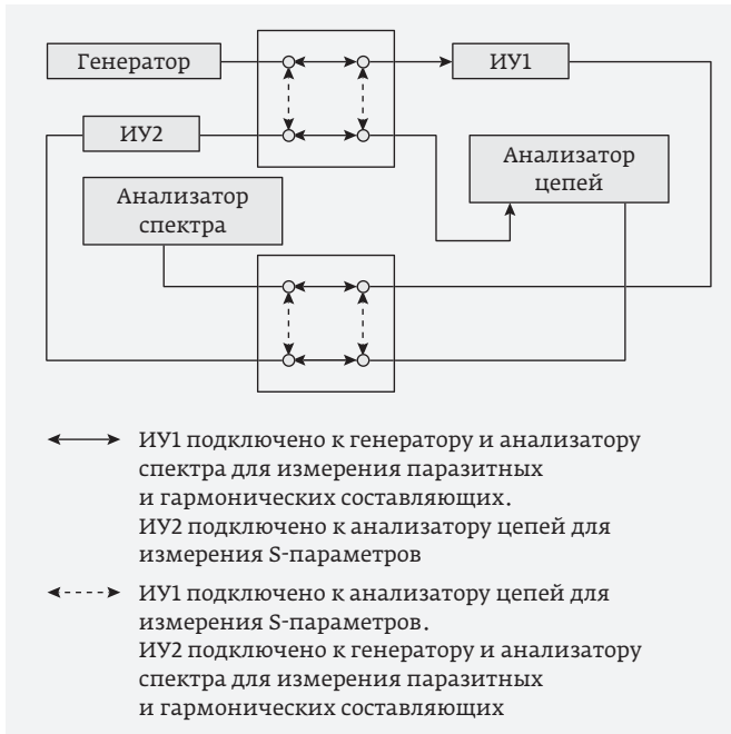
Рис. 29. Стенд для измерения S-параметров, паразитных и гармонических составляющих испытуемых устройств ИУ1 и ИУ2
