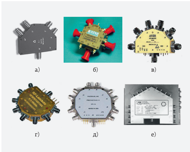
Рис. 26. Конструкции многопозиционных переключателей, отличные от приведенных на рис. 21 и 22: а – SP4Т (140-F106, RH Laboratories); б – SP4Т (S4317D, ATM), в – SP6Т (A35-MH134, AKON); г – SP8Т (RFSP8TA0118G, RF-Lambda); д – SP10Т (PSW10-0119-391-11, Paciwave); е – SP16Т (SWN-16TDA-HM-ARG, AMC)
