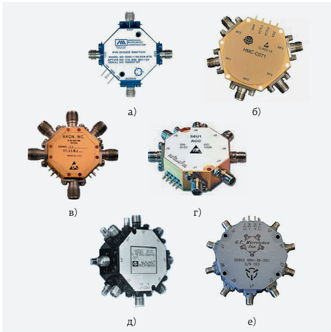
Рис. 22. Конструкции многопозиционных переключателей в квазидисковых корпусах: а – SP3Т (SWN-1140-3D, AMC); б – SP4Т (HMC-C071, Analog Devices); в – SP5Т (A35-MX195, AKON); г – SP6Т (S6U1, Cobham Signal & Control Solutions); д – SP7Т (9170-500, Kratos); е – SP8Т (R8N-39-2BU, G. T. Microwave)
