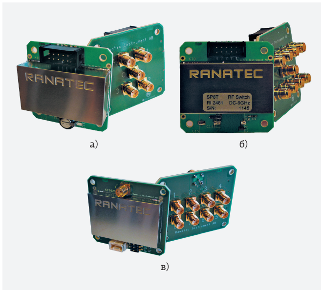
Рис. 27. Конструкции многопозиционных переключателей, выпускаемых компанией Ranatec: а – SP4Т (RI 2441); б – SP8Т (RI 2481); в – SP8Т (RI 2583)
