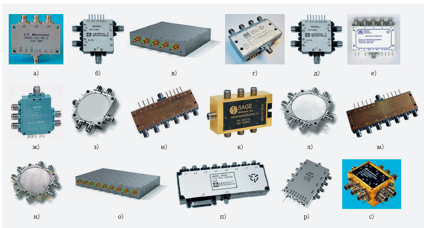
Рис. 21. Конструкции многопозиционных переключателей в прямоугольных корпусах: а, б – SP3Т (S3L-69-2, G. T. Microwave; E9130H, Kratos); в, г, д – SP4Т (CST-POE-SW04-1082, ETL; P4T-2G18-60-T-512-SFF, PMI; E9140H, Kratos); е, ж, з – SP5Т (MSN-5DT-05-STD, AMC; SS153DHTS, Narda Microwave; SW5-040120A14HM, Miteq); и, к, л – SP6Т (SW-SP6T-C1-1604, ETL; SK6-0232432520-KFKF-R1, Sage Millimeter; SW6-020180RN3HF, Miteq); м, н – SP7Т (SW-SP7T-C1-1605, ETL; SW7-005020AN3NM, Miteq); о, п, р, с – SP8Т (CST-POE-SW08-1083, ETL; F9180, Kratos; SW070-0S, R&K; CP8-29225040-01, Ducommun Technologies)
